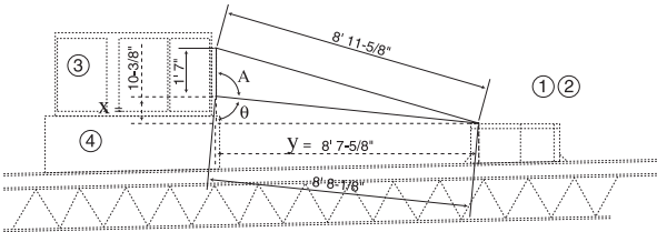
D1 — Elevation View
